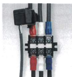
制御盤の中からでも無線伝送可能 (※環境により異なるが約50m程度)
